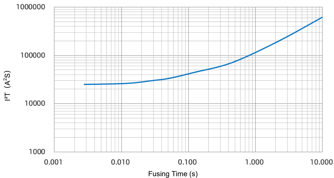
SKT 150 A I 2 t-t Curve
