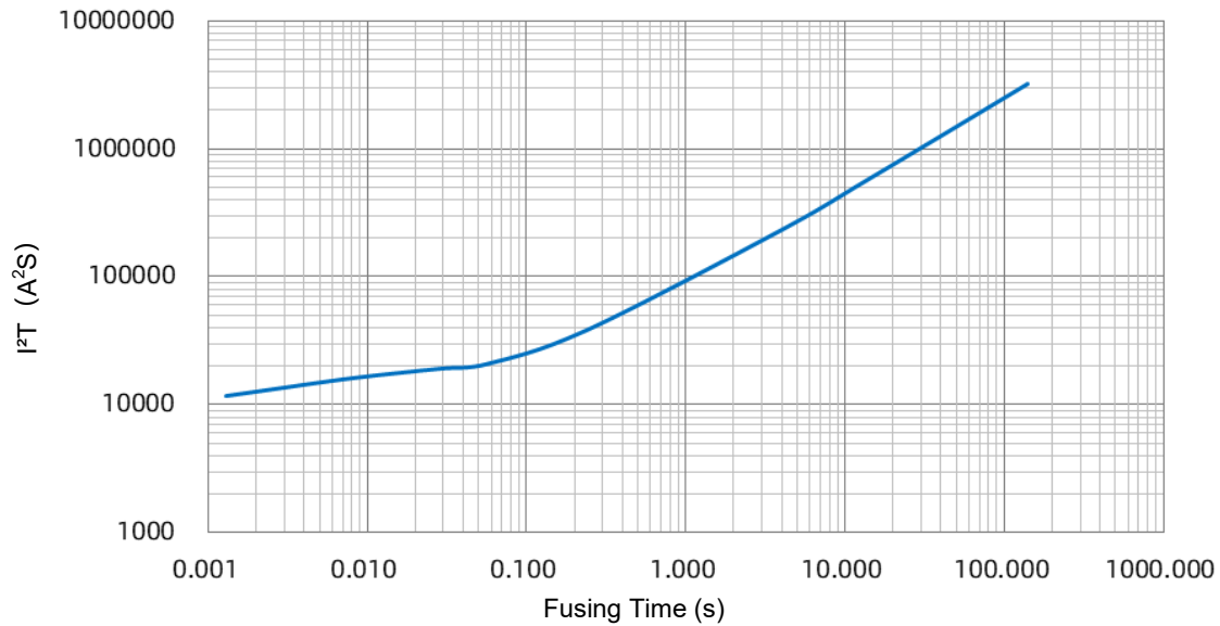
SKT 120 A I 2 t-t Curve
